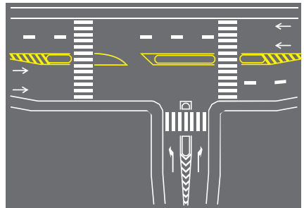
Ilhas de canalização e refúgio para pedestres
